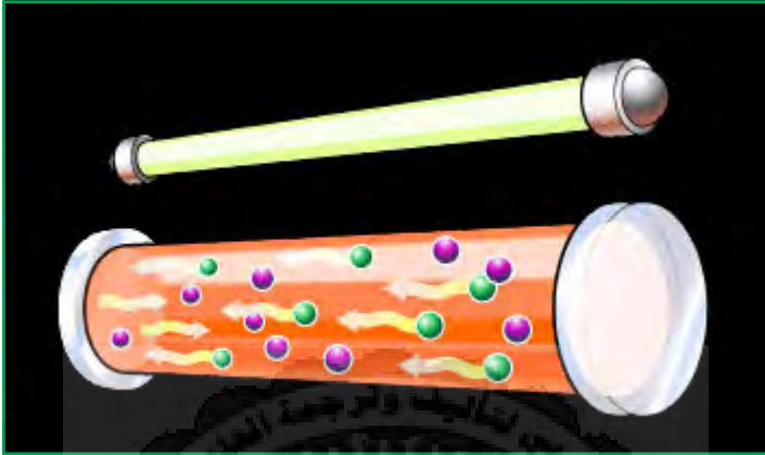
(الشكل 9): استحثاث الإلكترونات الأخرى لاطلاق الفوتونات
